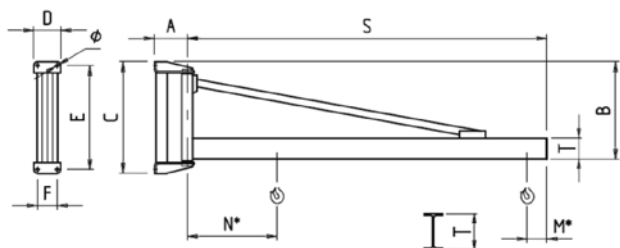
270° Gru a parete Rotazione 270°
