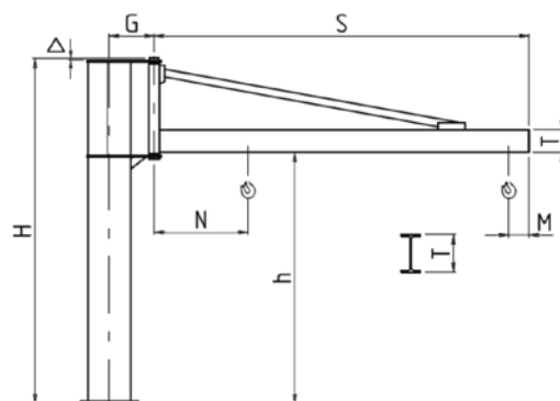
300° Gru a colonna Rotazione 300°
